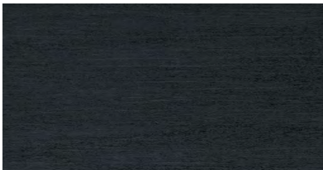
carbonio
