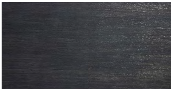
silicio
