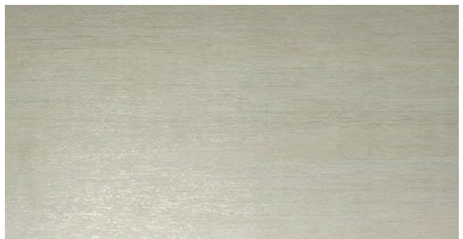
iridio
