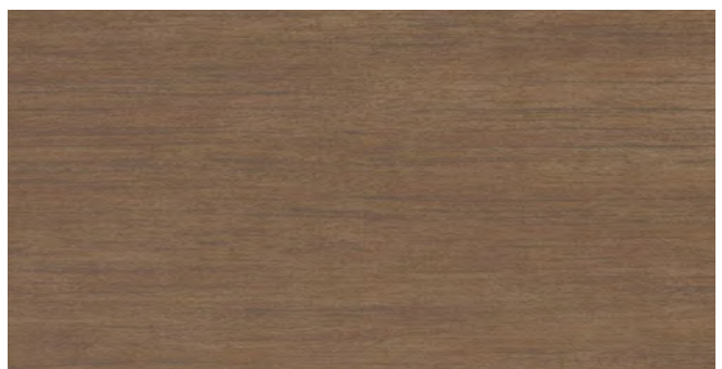
oro
