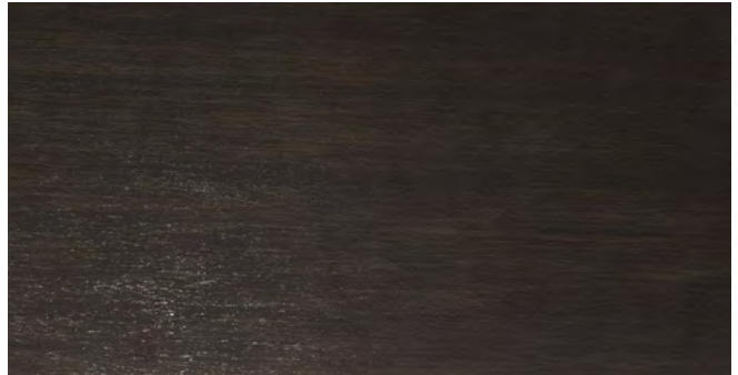
bronzo
