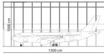
longitudinal section
